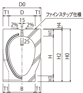
正面図
