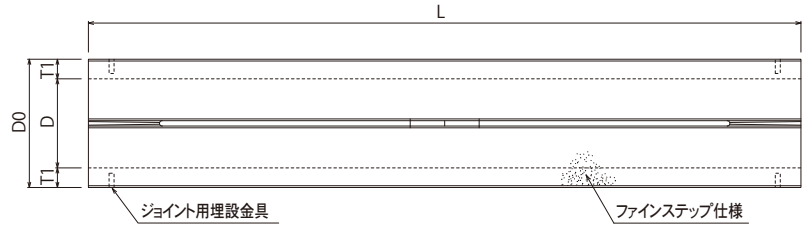
平面図
